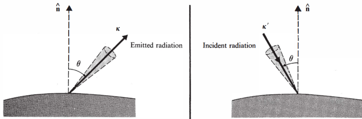
Figura 1: Diagrama que ilustra la emisión y absorción de radiaciones por un cuerpo.
