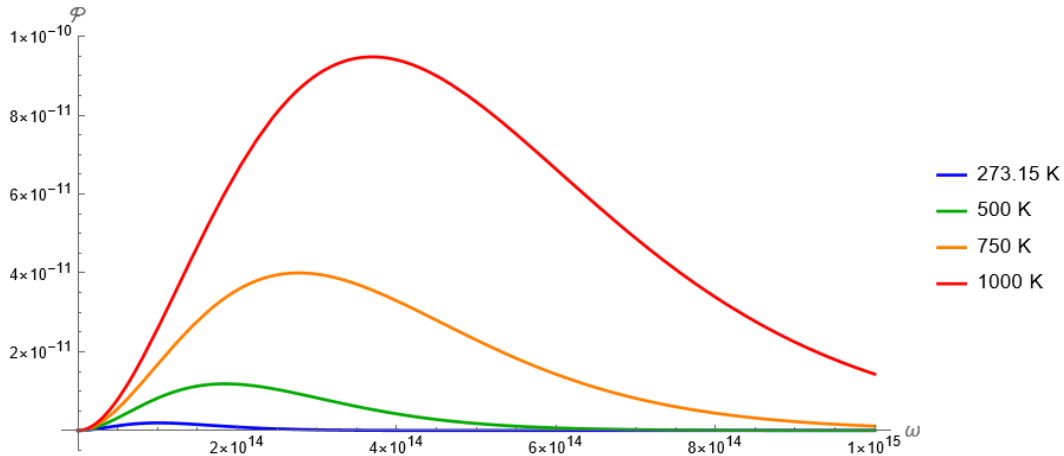
Figura 3: Espectro de emisión sobre frecuencia angular para 4 cuerpos negros a distinta temperatura.
